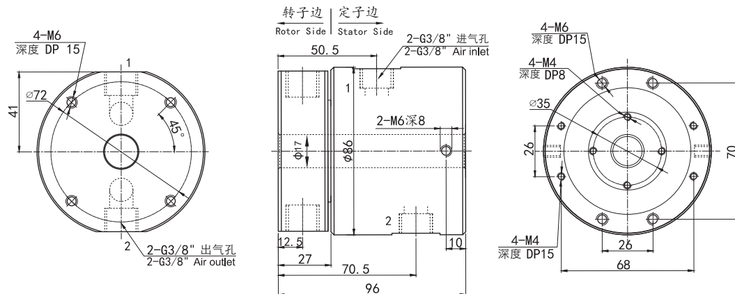
3002012 (2进2出，10~12mm气管，纯气动旋转接头) 尺寸图
