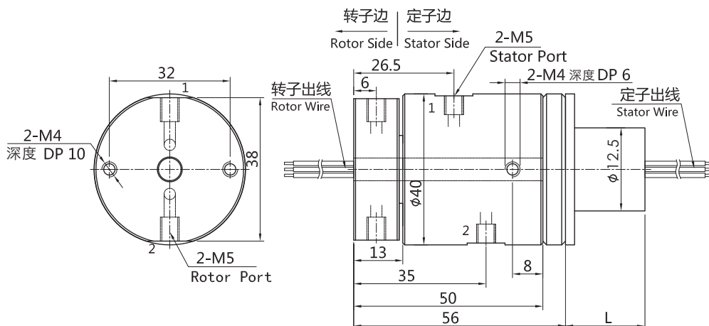
3002004 (2进2出,4mm气管)+6~36路信号/2A (适用于电磁阀与感应开关)
